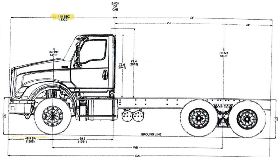
HX620_day_cab_6x4_isv
