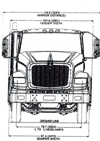
HX620_front
